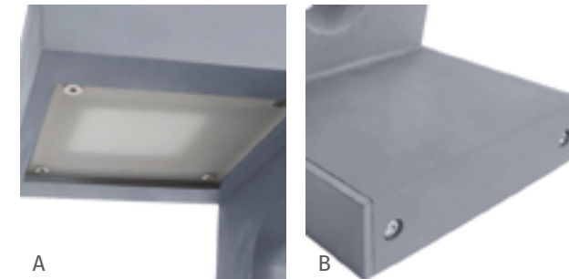
A: Vetro temperato acidato / Tempered etched glass / Geätztes gehärtetes Glas / Verre trempé satiné B: Coperchio per vano cablaggio e ancoraggio / Wiring and ground anchor compartment cover / Kabelanschlussraum und Bodenanker Sockel / Couvercle du compartiment électrique et de l'encrage au sol
