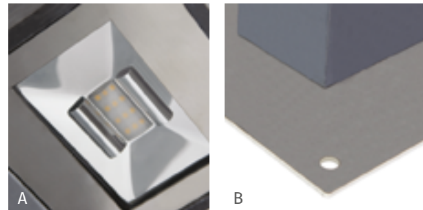
A: Piastra in acciaio inox satinato / Stainless satin steel Bracket / Halterung aus poliertem Edelstahl / Support en acier inoxydable satiné B: Base in acciaio / Steel Base / Fuß aus Stahl / Base en acier
